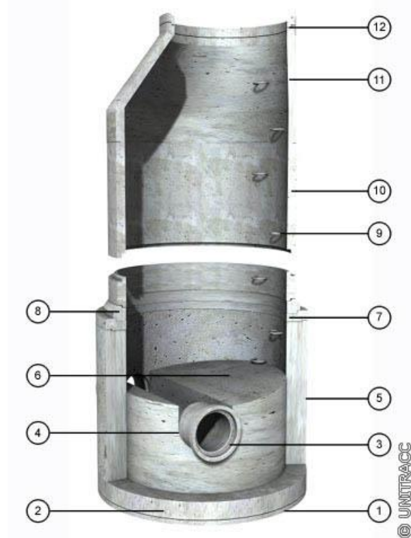
1000 Betonschacht Revision begehbar
